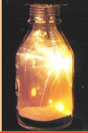
احتراق قطيلة الحديد في ثنائي الاوكسجين
