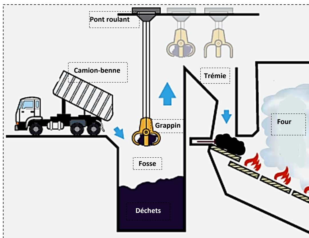
Fig. 1 : Schéma partiel d'une usine d'incinération de déchets
